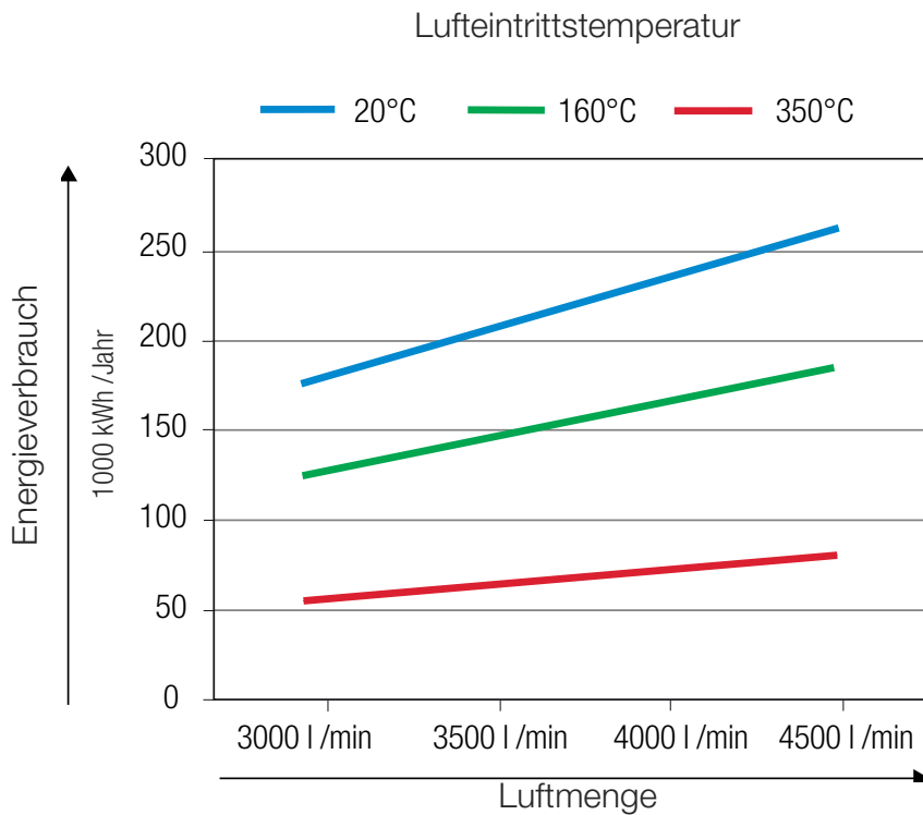
Stromverbrauch im 24-Stunden-Betrieb, an 250 Tagen/Jahr. Gut ersichtlich: Je höher die Lufteintrittstemperatur, desto niedriger der Energieverbrauch.
