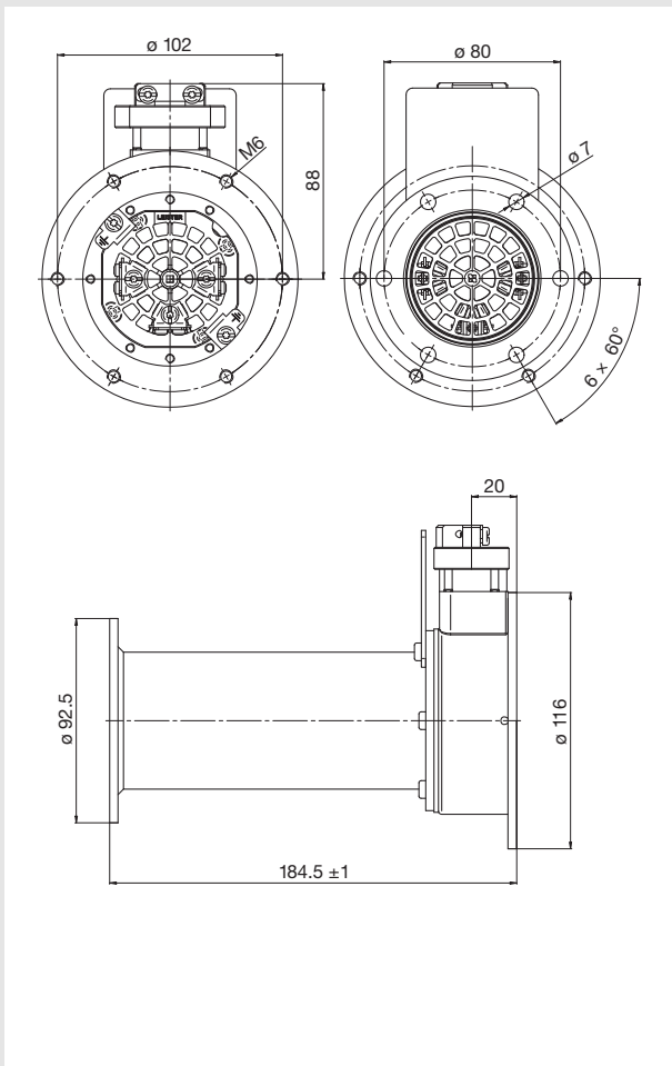
Einbaumassee LE 5000 DF-R in mm
